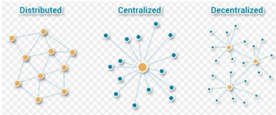
[그림3] 스마트컨트랙트
